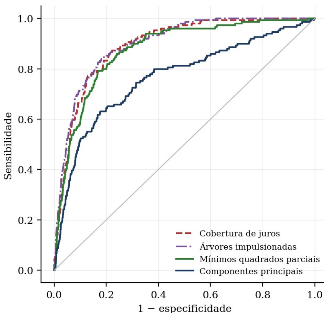
Figura 2 – Curvas ROC fora da amostra, horizonte de um ano
