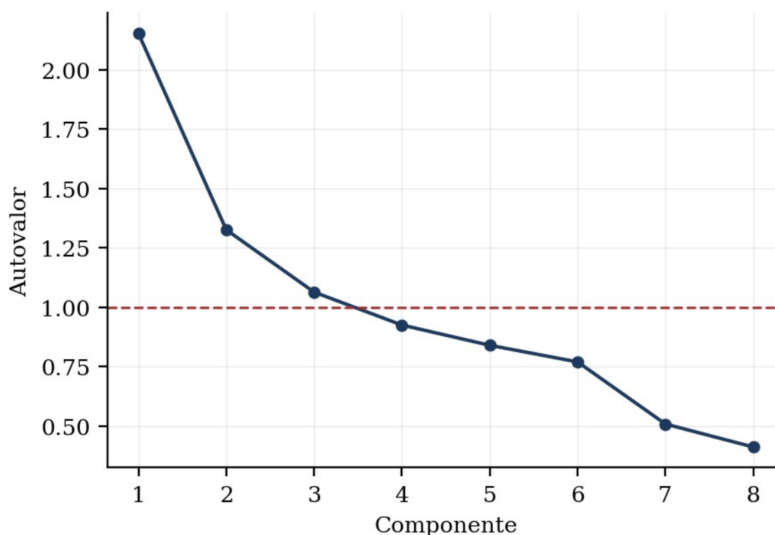
Figura 1 – Autovalores dos componentes principais
